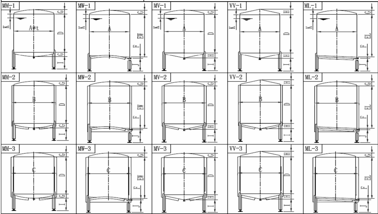
尺寸表(mm)
